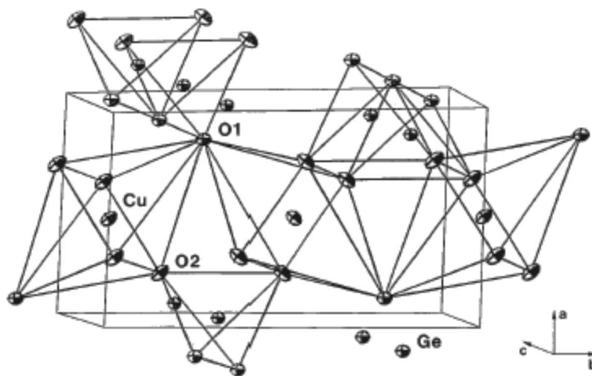
Рис. 2: Кристаллическая структура \text{CuGeO}_3 в высокотемпературной фазе (по данным работы [35]).
