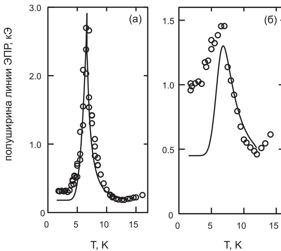
Рис. 6: Зависимость ширины линии ЭПР от температуры для образцов \text{Cu}_{1-x}\text{Ni}_x\text{GeO}_3 с x=0.2\% (а) и x=0.8\% (б). Сплошные линии - теоретический расчет [36].
