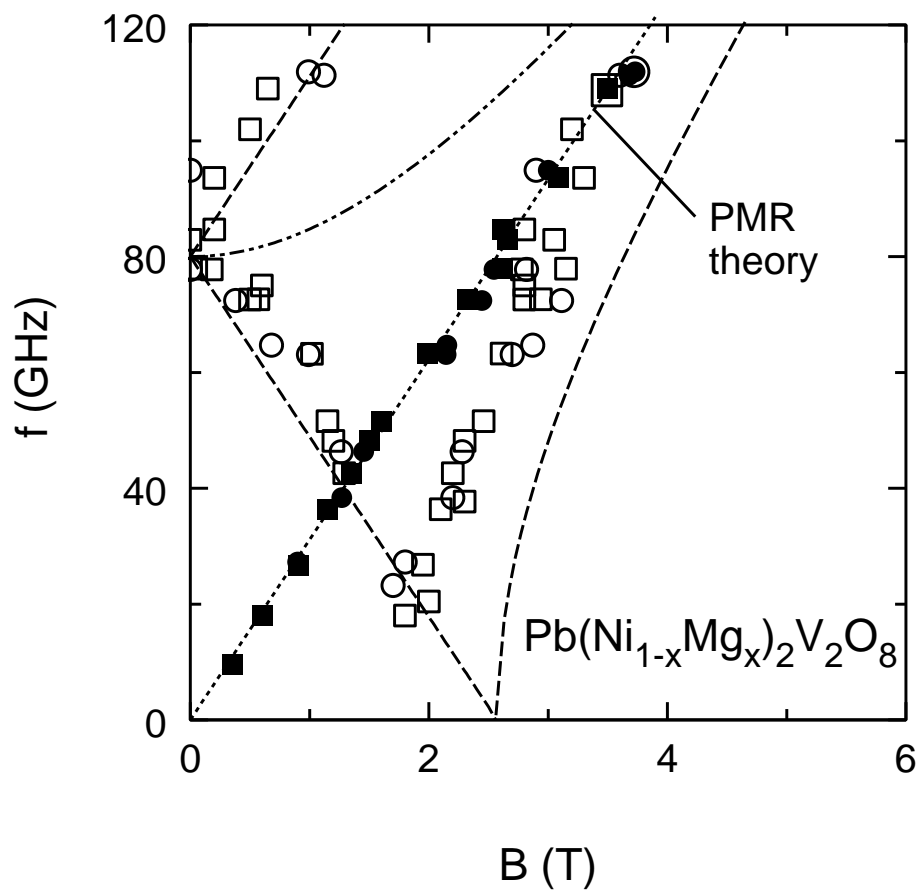
Рис. 10: Зависимость резонансной частоты от магнитного поля керамических образцов \text{Pb}(\text{Ni}_{1-x}\text{Mg}_x)_2\text{V}_2\text{O}_8 в парамагнитной фазе ( T=5 К, черные символы) и в упорядоченной фазе ( T=1.3 К, неокрашенные символы) [50]: x = 0.04 - кружки; x = 0.06 - квадраты. Значение пунктирных и точечных линий приведено в тексте.
