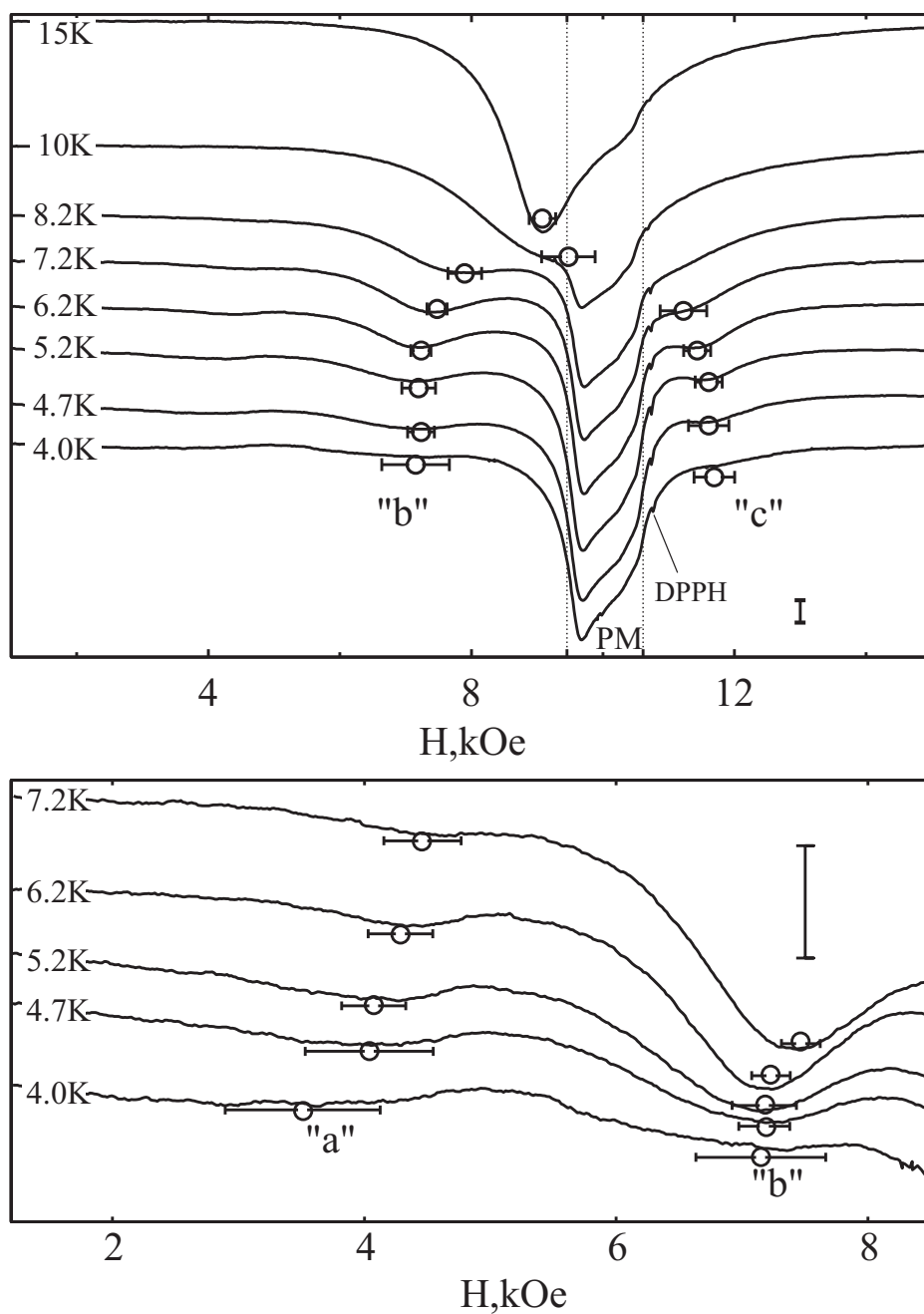
Рис. 23: Линии магнитного резонанса термоактивированных триплетных возбуждений в димерном магнетике \text{TiCuCl}_3 ("a", "b", "c"). РМ - линия магнитного резонанса паразитного гидратного соединения, загрязняющего поверхность образца [70].
