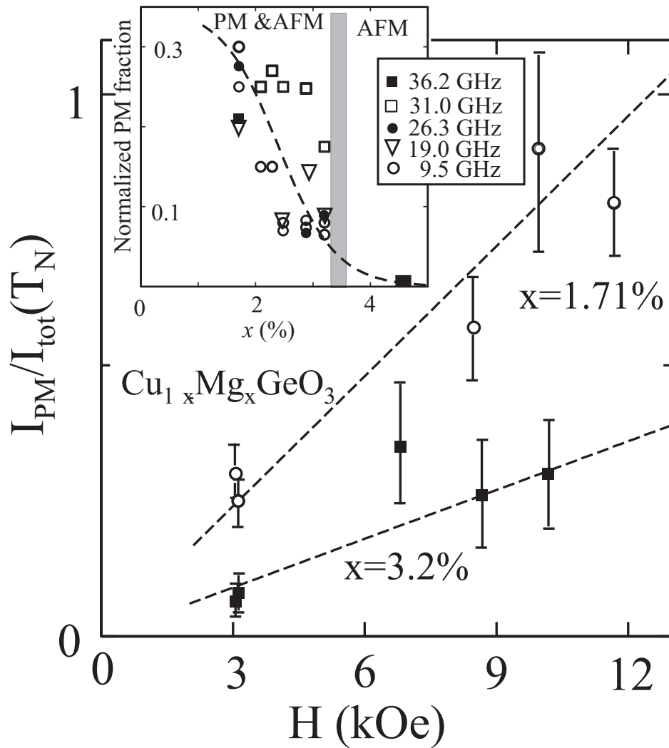
Рис. 21: Зависимость концентрации парамагнитной фазы от магнитного поля при температуре, близкой к точке Нееля со стороны антиферромагнитной фазы. На вставке - зависимость доли парамагнитной фракции от концентрации примесей [44].
