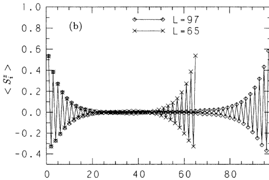
Рис. 1: Спиновая структура фрагмента халдейновской спиновой цепочки с открытыми граничными условиями для нечетного числа спинов и полной проекции S_{tot}^z = 1 . (из работы [11]). По горизонтальной оси отложен номер магнитного иона во фрагменте цепочки.
