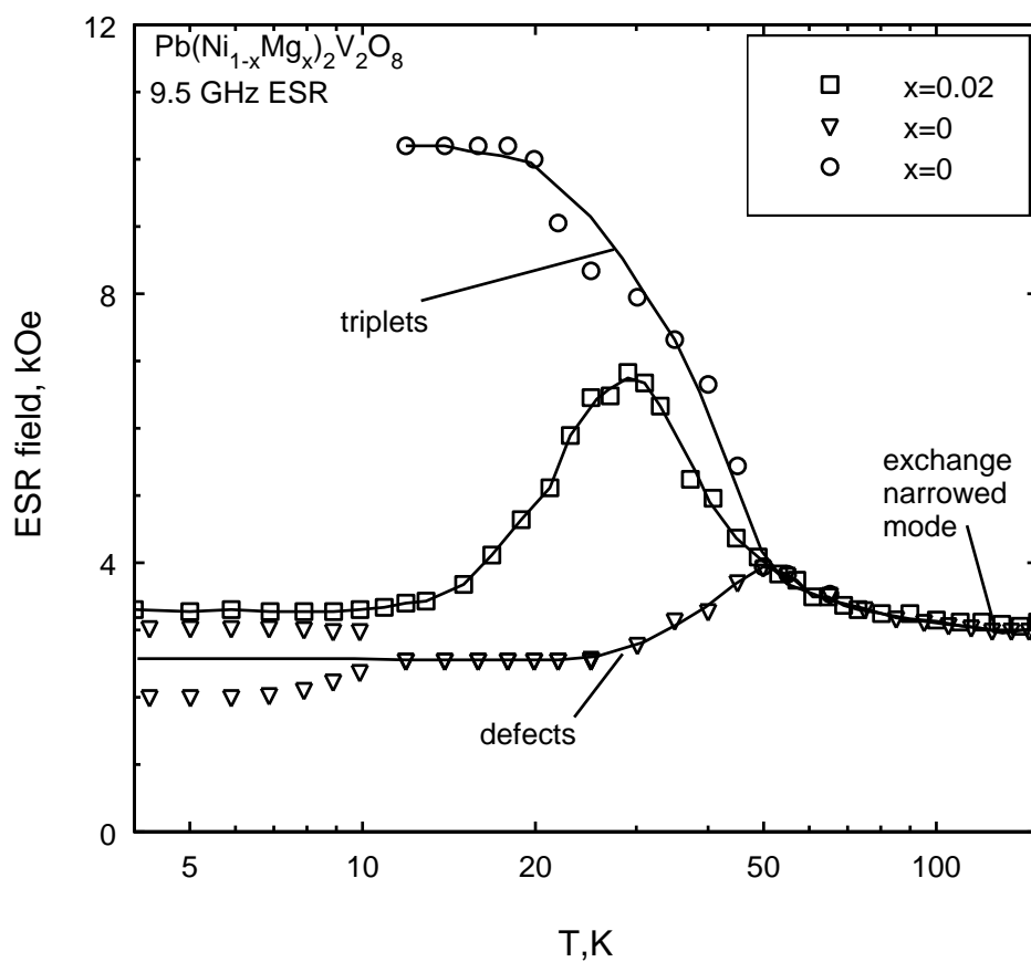
Рис. 11: Зависимость поля магнитного резонанса от температуры для различных видов спиновой прецессии в допированных образцах халдейновского магнетика \text{PbNi}_2\text{V}_2\text{O}_8 . [55]
