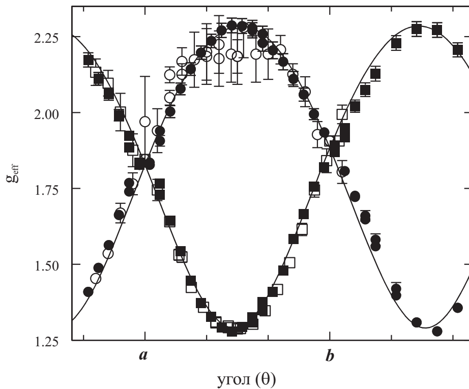
Рис. 7: Угловая зависимость эффективного g -фактора компонент линии поглощения в образце \text{Sr}_{1-x}\text{Ni}_x\text{GeO}_3 с концентрацией примеси x=0.2\% , полученная при вращении магнитного поля в плоскости (ab) . \blacksquare, \bullet — данные полученные на частоте 9.5 ГГц; \circ, \square — на частоте 36 ГГц.
