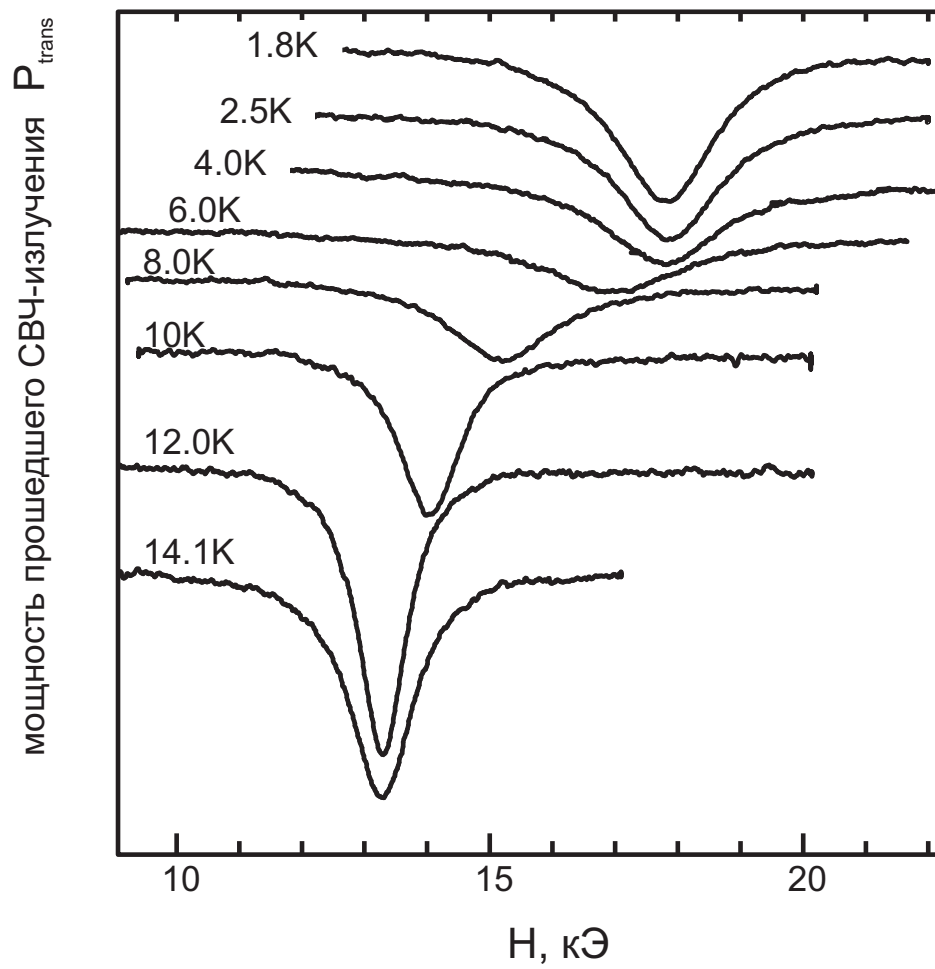
Рис. 4: Эволюция формы линии магнитного резонанса образца \text{Cu}_{0.992}\text{Ni}_{0.008}\text{GeO}_3 при изменении температуры [36]. f=36 ГГц, H||c .
