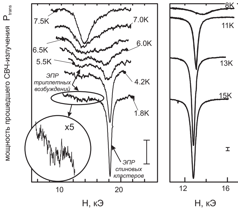
Рис. 3: Эволюция формы линии резонансного поглощения образца \text{Cu}_{0.998}\text{Ni}_{0.002}\text{GeO}_3 при изменении температуры [36]. f=36 ГГц, H||c . Вертикальные отрезки на левой и правой панелях соответствуют одинаковой величине поглощения.
