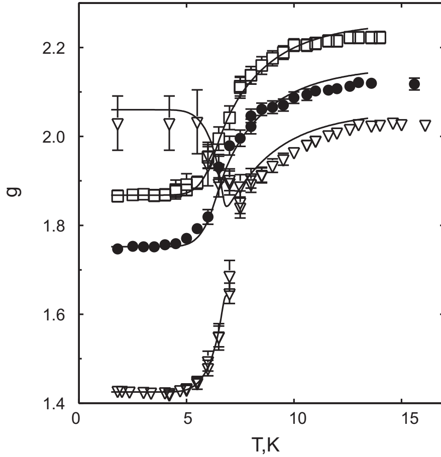
Рис. 5: Зависимость g -фактора от температуры для образца \text{Cu}_{0.998}\text{Ni}_{0.002}\text{GeO}_3 [36]. точки - H \parallel a , квадратики - H \parallel b , треугольники H \parallel c , сплошные линии - теоретический расчет на основе модели обменного сужения.
