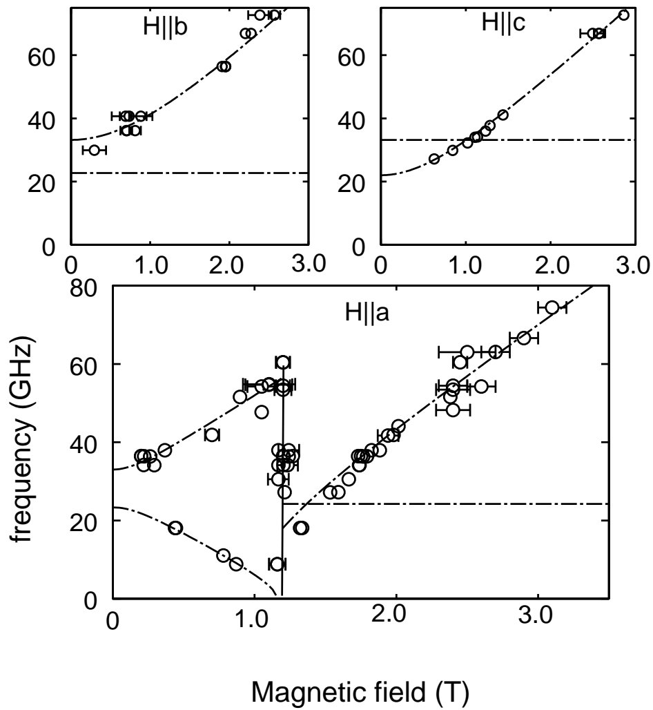
Рис. 12: Зависимости резонансных частот спиновых колебаний в упорядоченной фазе образца \text{Cu}_{1-x}\text{Ni}_x\text{GeO}_3 , x = 0.032 , T = 1.8 К [45].
