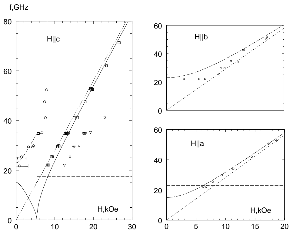
Рис. 14: Зависимости резонансных частот спиновых колебаний в упорядоченной фазе образца \text{Cu}_{1-x}\text{Zn}_x\text{GeO}_3 , x = 0.04 , T = 1.4 K [60].
