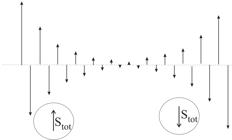
Рис. 20: Схематическое изображение областей локального антиферромагнитного порядка вблизи концов оборванных примесью спиновых цепочек и результирующих магнитных моментов этих областей.
