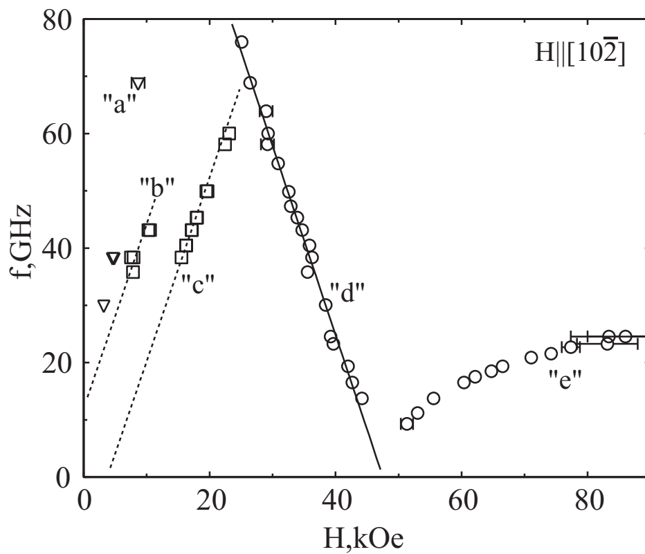
Рис. 24: Спектр магнитного резонанса низколежащих триплетных возбуждений ("a", "b", "c"), зависимость спиновой щели от магнитного поля ("d"), частота спиновых колебаний в упорядоченной фазе ("e") [70].
