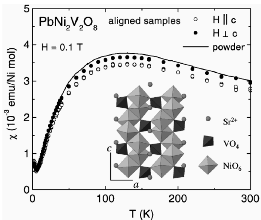
Рис. 8: Температурная зависимость магнитной восприимчивости \text{PbNi}_2\text{V}_2\text{O}_8 . На вставке: схема кристаллической структуры (\text{Pb}/\text{Sr})\text{Ni}_2\text{V}_2\text{O}_8 . Из работы [33]
