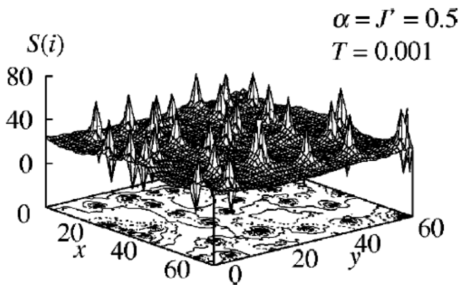
Рис. 19: Результат численного моделирования [63] задачи о средних значениях проекций спинов в узлах двумерной сетки из димеризованных цепочек с межцепочечным взаимодействием.
