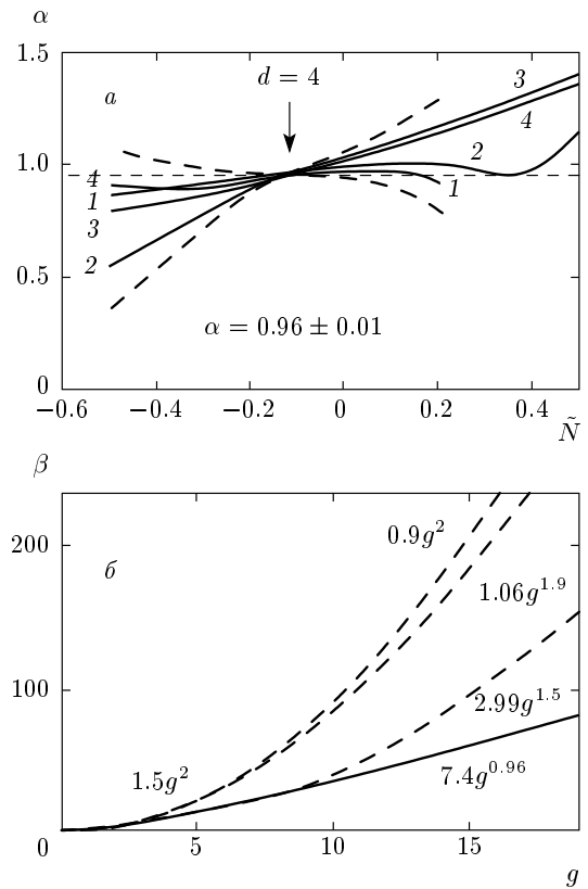
Рис. 1. Результаты для четырехмерной теории \varphi^4 : a — зависимость показателя \alpha от \tilde{N} (его различные оценки описаны в [4]); b — общий вид функции Гелл-Манна–Лоу согласно [4] (сплошная кривая) и результаты других авторов — пунктирные кривые сверху вниз соответствуют результатам работ [16–18]
