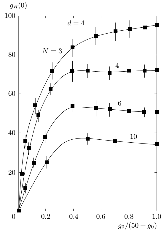
Рис. 7. Зависимость перенормированного заряда g_R(0) , взятого при нулевых импульсах, от затравочного заряда g_0 , относящегося к межатомному расстоянию a_0 , в четырехмерной теории \varphi^4 при фиксированных значениях N a_0 и m , но различном числе N^4 узлов решетки (согласно работе [51])
